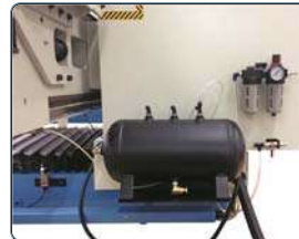
Réservoir d'air intégré et filtreur régulateur lubrificateur
