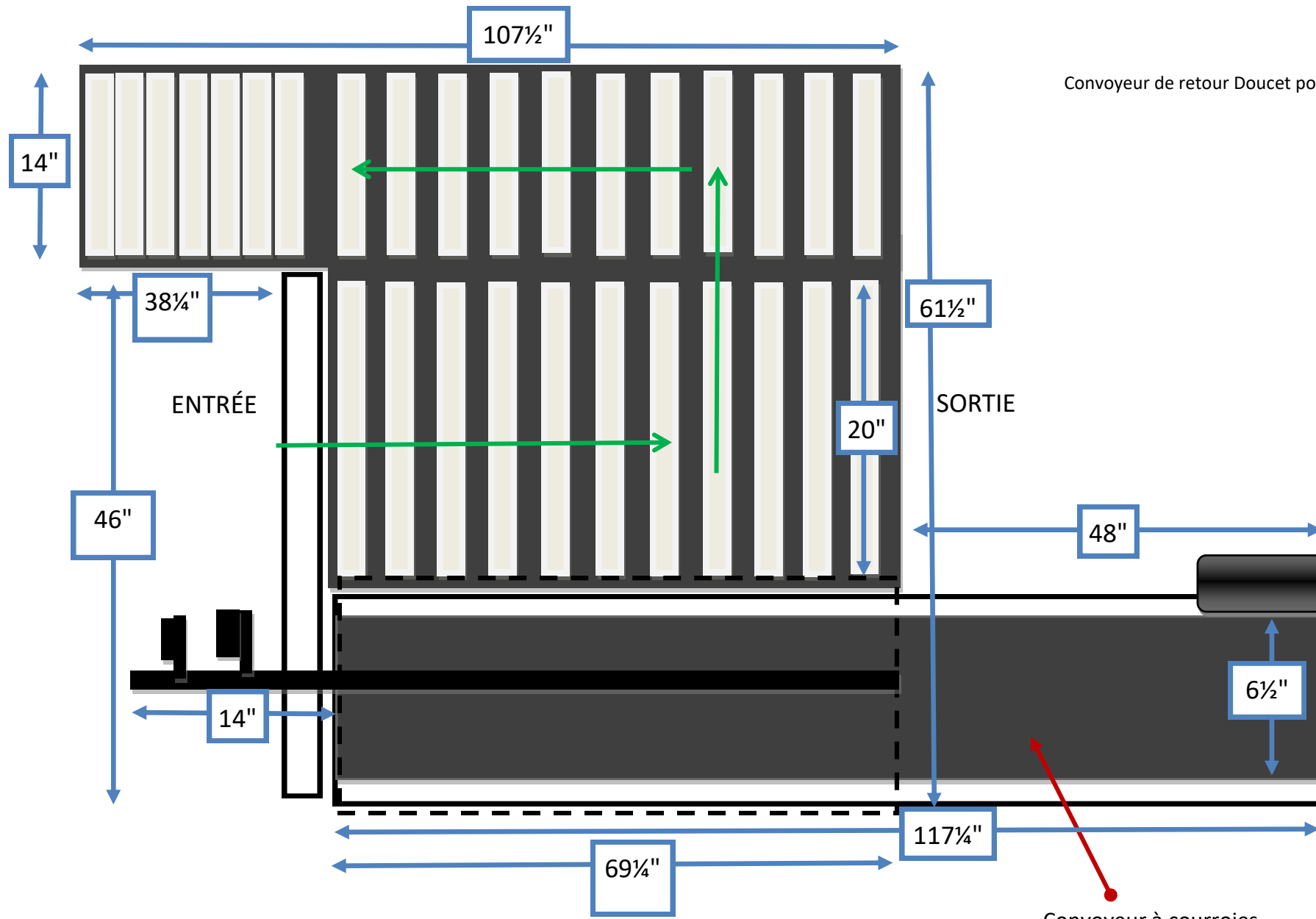
Convoyeur à courroies Extraction bon bois et rebuts
